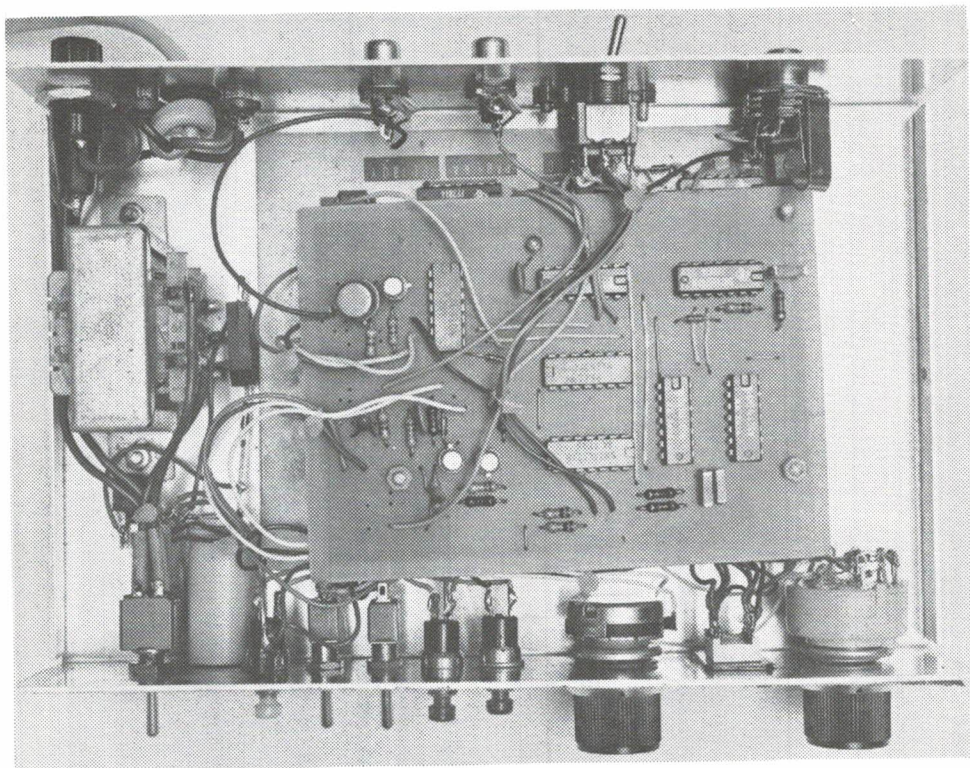
Het inwendige van de STIVECO momry-keyer. De beide printen zijn boven elkaar gemonteerd om ruimte te sparen.
