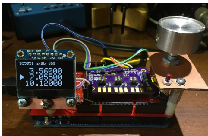
Foto: 3 bands VFO met de Si5351 als hart van de schakeling.
